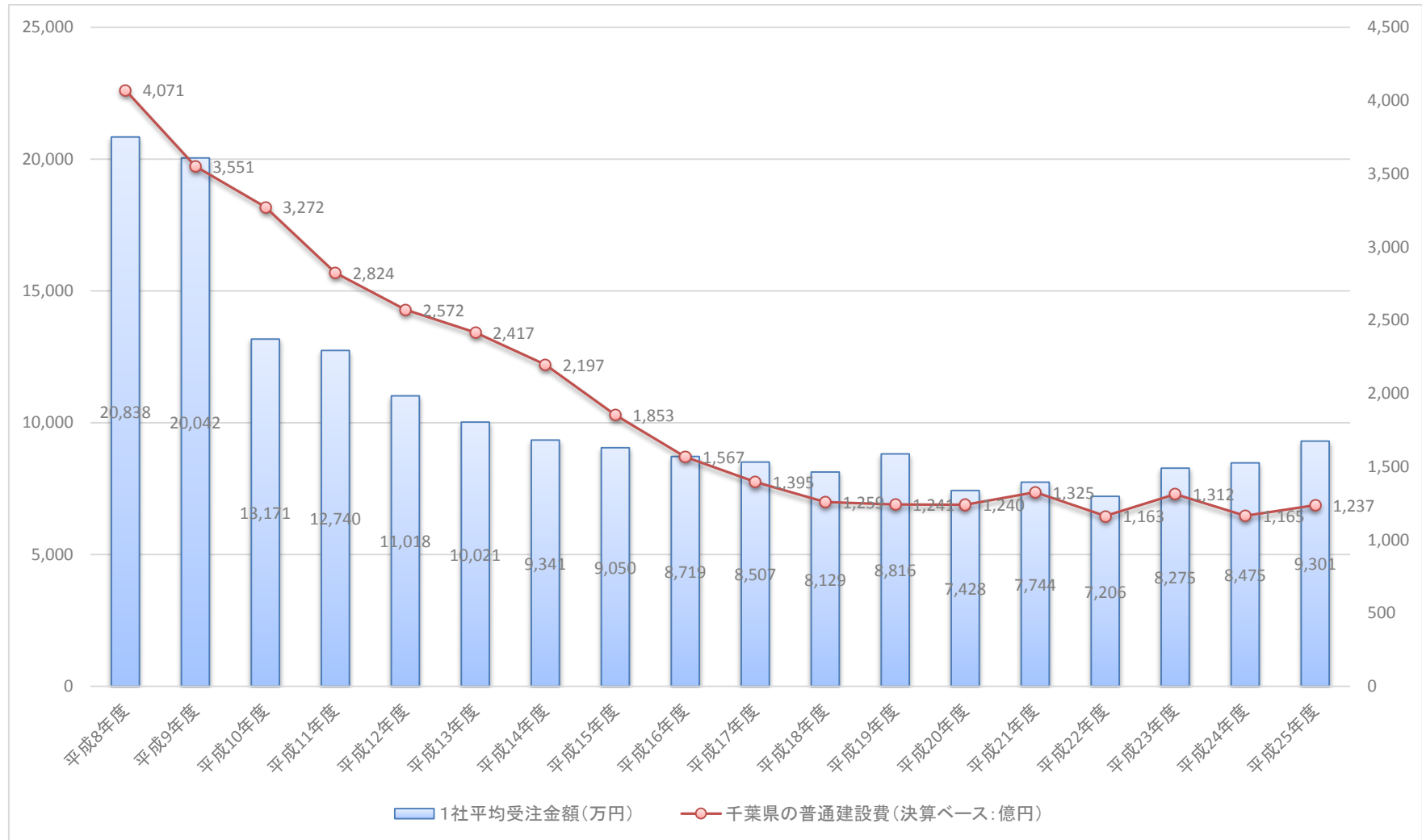
【グラフ2】 県の普通建設費と会員1社当り平均年間受注金額の推移(過去18年間)
